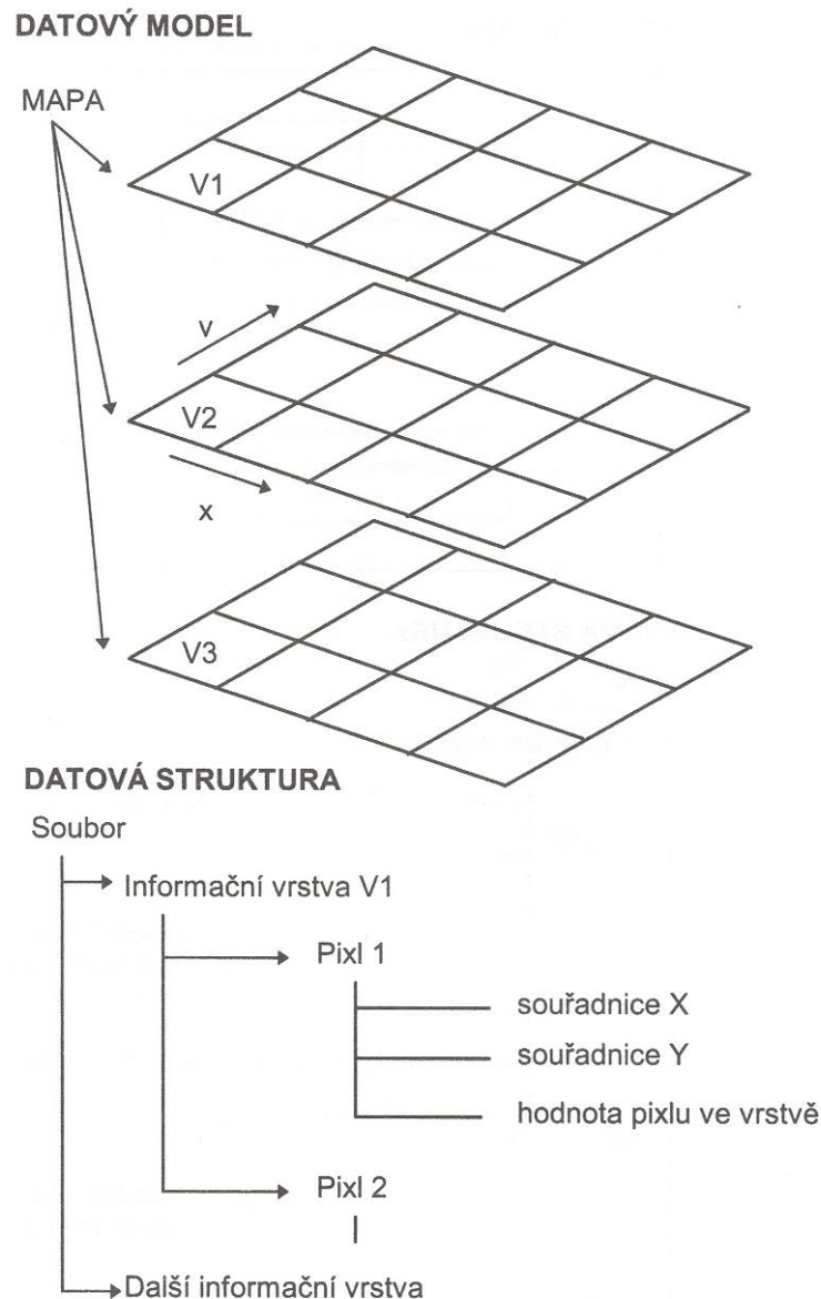
Obr. 9.4. Rastrový datový model a struktura (Voženílek, 1998).
