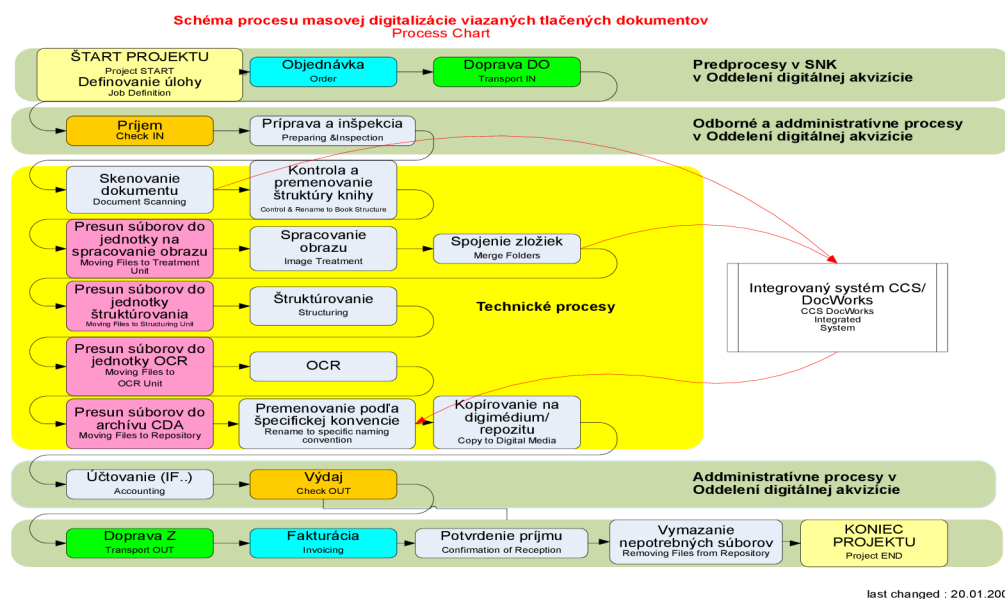
Obrázok 5 Schéma procesov v projekte digitalizácie menšieho rozsahu aj s prihliadnutím komerčné využitiu
