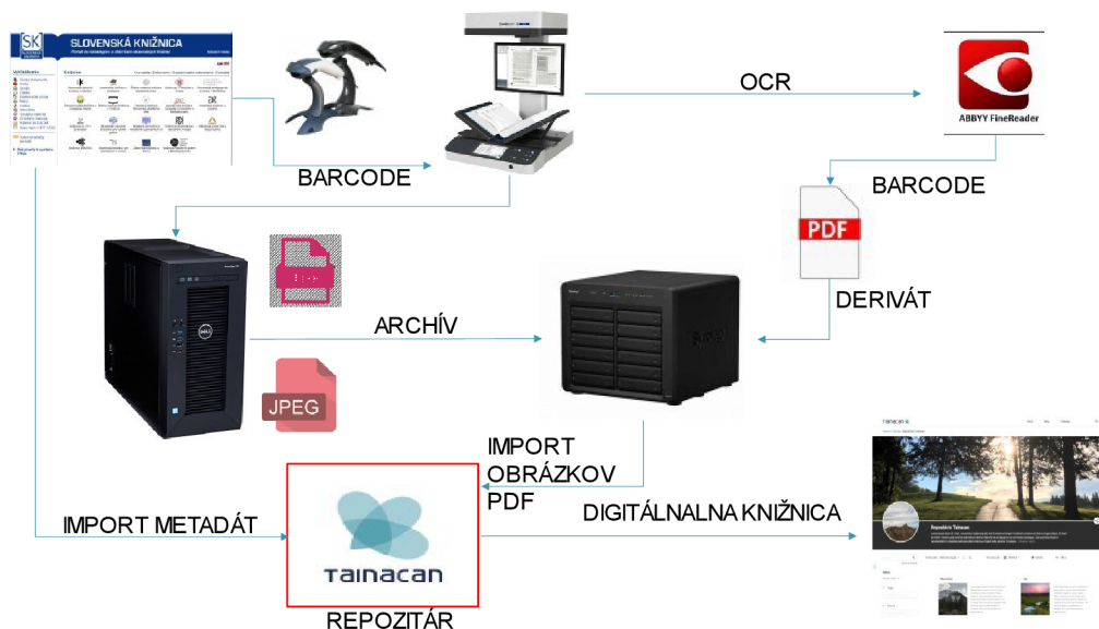
Obrázok 4 Schéma malej digitalizácie v knižnici
