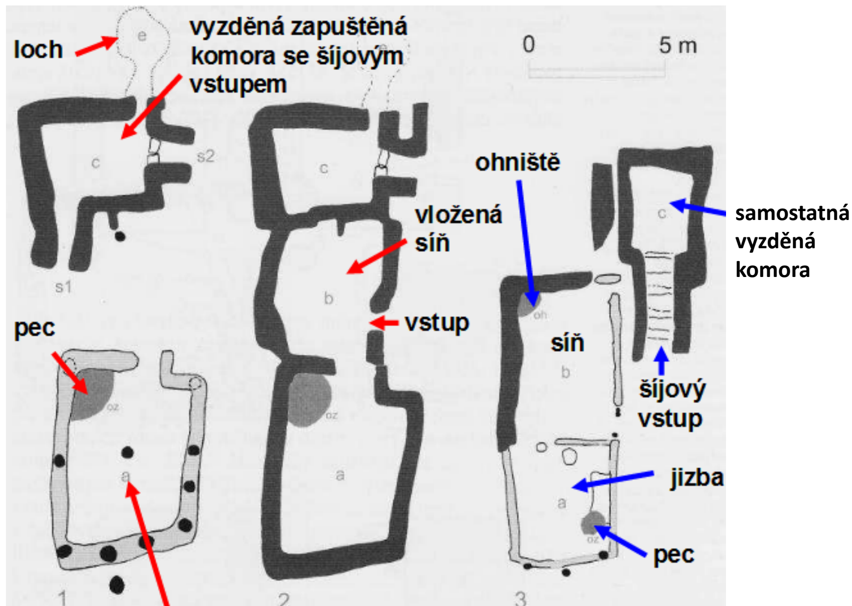
samostatná jizba sloupové konstrukce
