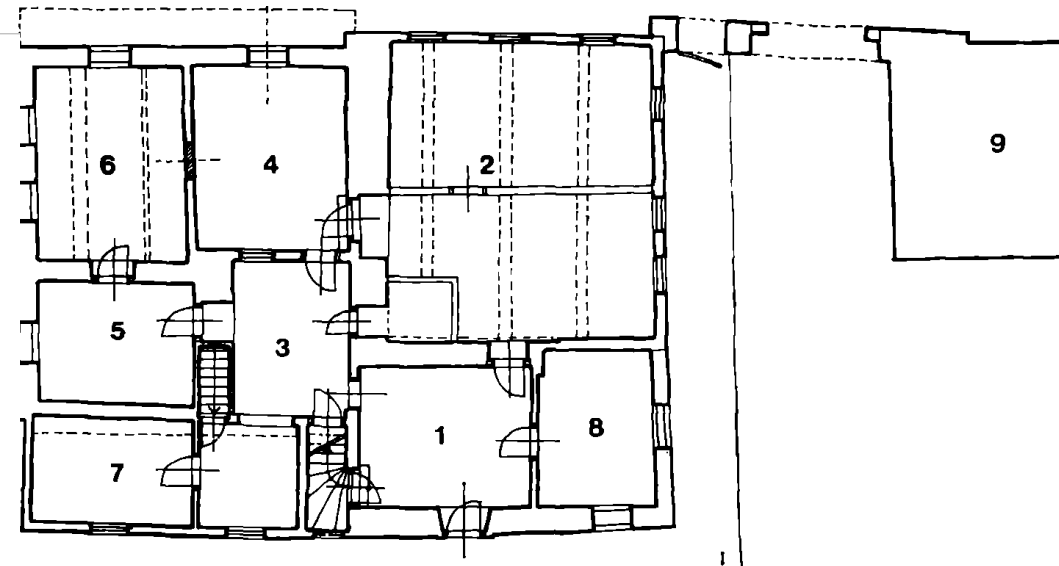
Obr. 2. Všeň čp. 14 (okr. Semily), půdorys přízemí. 1, 8, 7 – síň, světnička a komora v mladším zděném bočním traktu, 2 – jizba s novodobou příčkou, 3, 4 – síň, 5, 6 – komory, 9 – přízemní sroubek s dvěma komorami.
