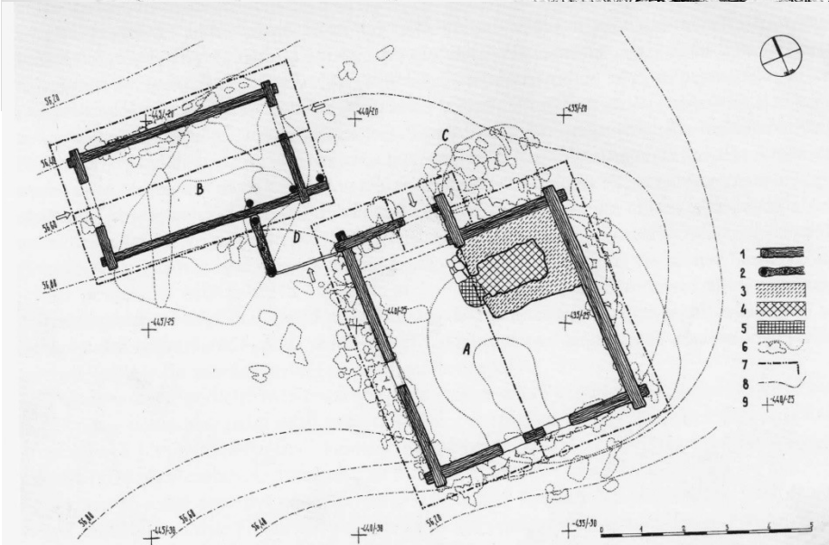
Obr. 19 Rekonstrukce půdorysu mladší fáze U IV, 1-roubená obvodová stěna, 2-oplétaná stěna, 3-zdivo pece, 4-prostor pece, 5-ohniště, 6-nálezová situace, 7-hrany a lomy možného zastřešení, 8-vrstevnice po dvaceti centimetrech, 9-body pětmetrové čtvercové sítě, A-jizba, B-komora, C-dlažba, D-uzavření usedlosti.
