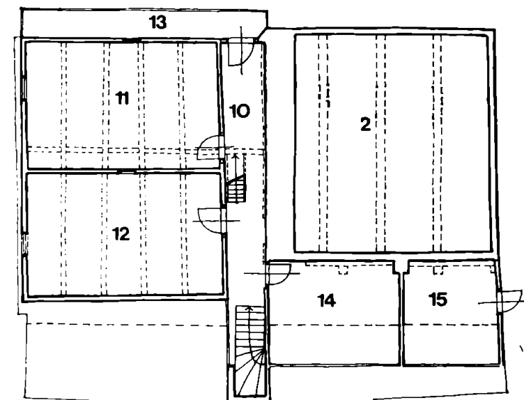
Obr. 3. Všeň čp. 14 (okr. Semily), půdorys patra. 2 – jizba, 10 – horní síň, 11, 12 – komory, 13 – pavlač, 14, 15 – mladší komory.
