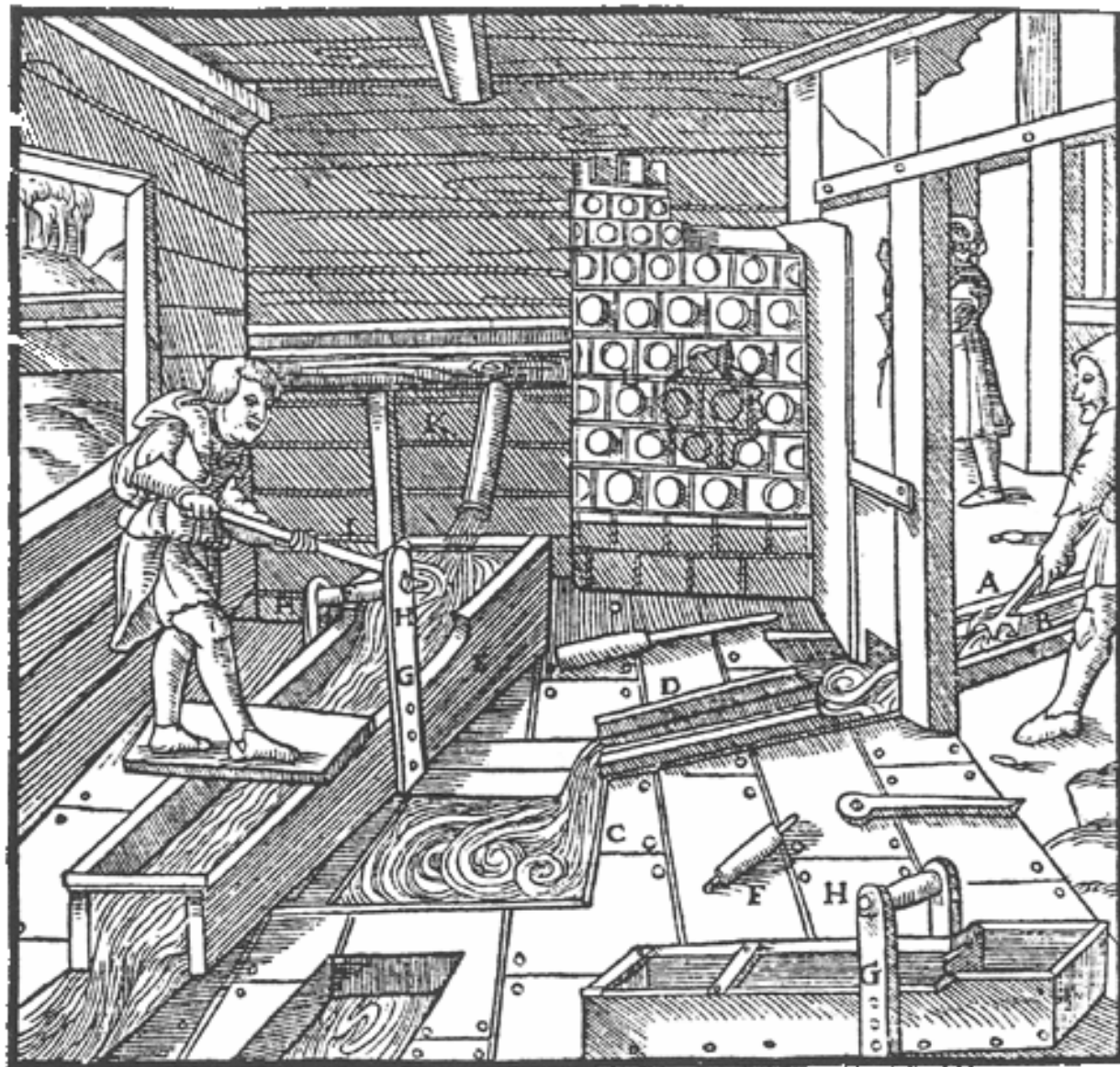
Dřevoryty, "De re metallica", Georg Agricola, 1556.
