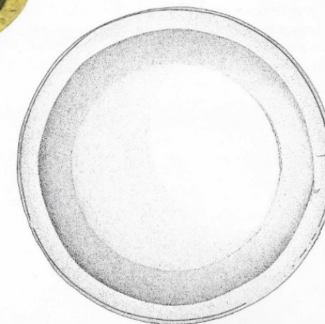
Opava, ulice Mezi Trhy (vnitroblok Drůbeží trh) první polovina 15. století výška: 6 cm, průměr: 19 cm (okraj), 17 cm (dno) mosaz (cca 83,5 % mědi; 15,3 % zinku; 0,8 % olova) NPÚ, ÚOP v Ostravě, inv. č. 50/05-142/510 foto T. Ott, kresba I. Tichá
