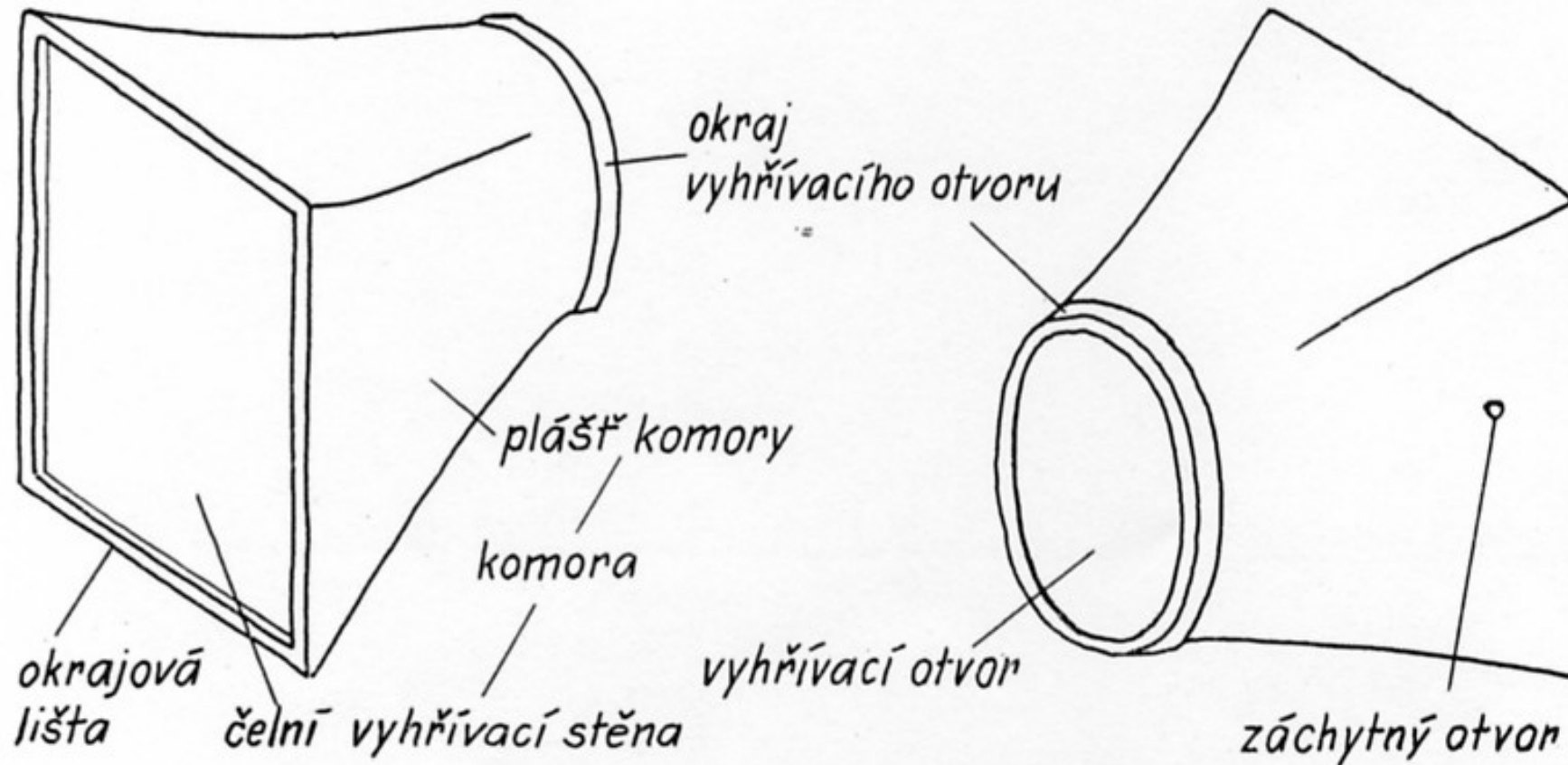
Obr. 14. Schema nejběžnějšího komorového kachle (s komorou kuželovitou).
