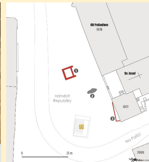
Středověká vápenka se vsázkou vápenců.
