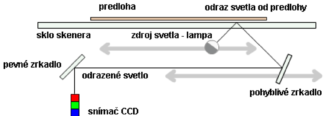
Obrázok 1 Schéma procesu snímania skenerom
