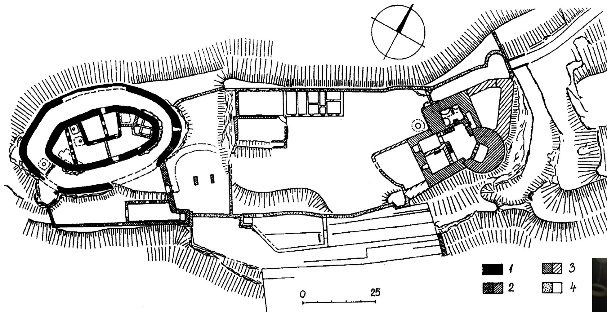
Obr. 290: Nový Hrádek — vývojové schéma hradu. Legenda: 1 - 14. století, 2 - první polovina 15. století, 3 - druhá polovina 15. až začátek 16. století, 4 - zbytek 16. století a pozdější.
