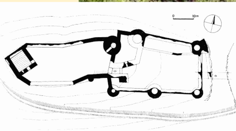
Týřov: 1973 a 1976-84 – výzkum T. Durdíka Dolní hrad – 6 flankovacích věží o průměru: 5,8 – 7,3 m
