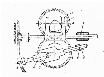
Obr. 40. Vyplnění perforačního otvoru filmu jističím čepem. Po stranách je váleček, jistič je ve svislém směru.
