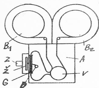
Obr. 18. Princip filmové kamery s filmem v jedné rovině. A - skříň kamery, B 1 -B 2 - zásobníky filmové suroviny, D 1 -D 2 - strhovací zařízení, V - transportní ozubený bubínek, G - filmový kanál, Z - objektiv, Ž - závěrka kamery.
