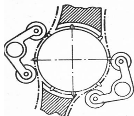
Obr. 44. U transportního bubínku bývá též shazovač filmu.
