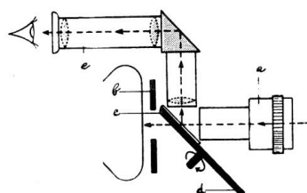
Obr. 75. Princip zosměřovací lupy se zrcadlovou závěrkou. a - objektiv, b - filmový kanál, c - závěrka se zrcátkem, d - protěží štát závěrky a výhledem k osivku filmu, e - zosměřovací lupy s optickou lomenou osou.
