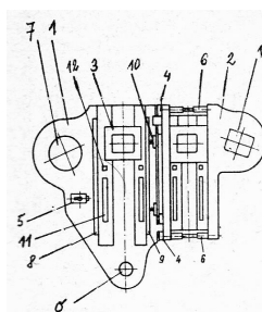
Obr. 41. Filmový kanál kamery Super Parvo Debrle: 1 - základní deska, 2 - dvíčka, 3 - kývavý rámeček, 4 - závěsy (panty), 5 - zámeček, 6 - dvě kladlíčky, 7 - matnice, 8 - nepokrytá vodící lišta, 9 - pohyblivá vodící lišta, 10 - spirálové pružiny lišty, 11 - výřez pro drápák, 12 - výřezy pro lišty šepy, 13 - výřez osazující obraz na matnici.
