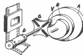
Obr. 20. Maltézský kříž. A - setrvačnick, B - vodící disk, V - kolík, G - maltézský kříž, D - ozubený bubínek
