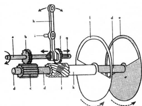
Obr. 44. U transportního bubínku bývá též shazovač filmu.
