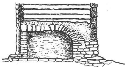
ŘEZ I-I'
