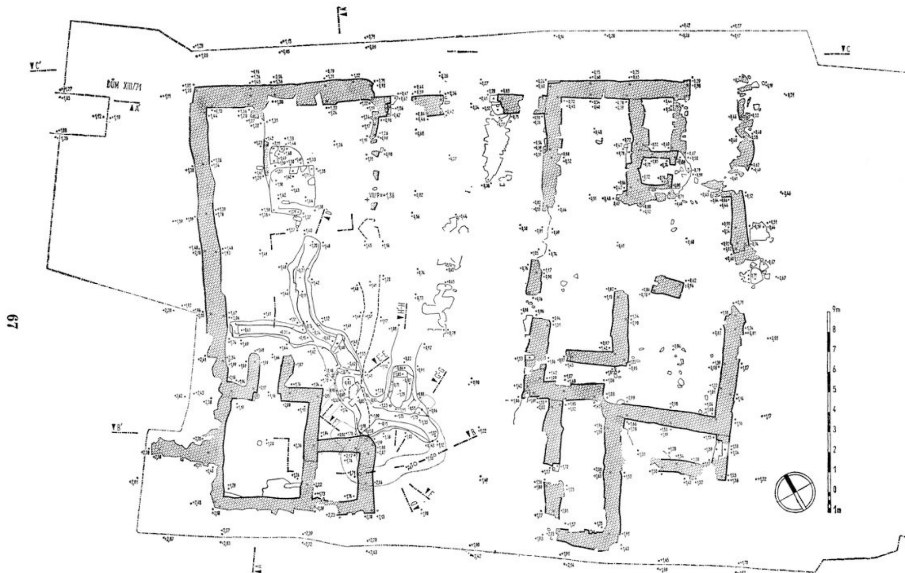
62a. Pfaffenschlag. Půdorys domů IX a X
