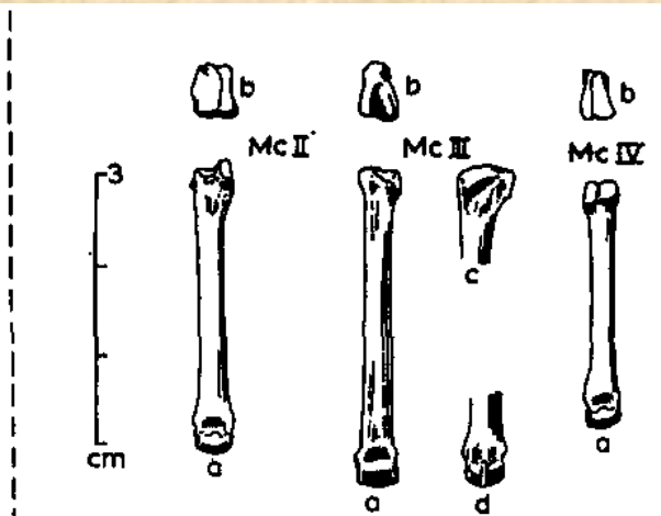
LEPUS
