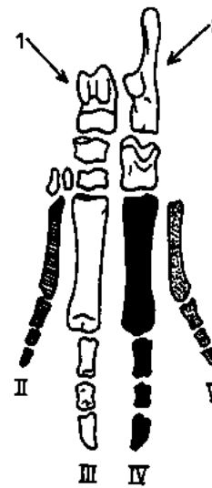
SUS post.
