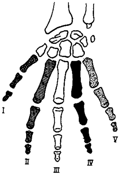
HOMO ant.
