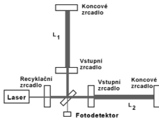
Schéma soustavy LIGO
