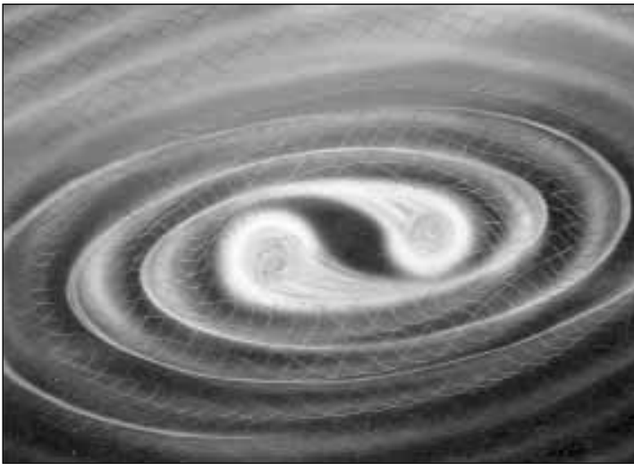
Gravitační vlna vytvářená dvojicí neutronových hvězd
