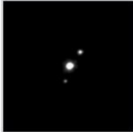
Haumea (2004)
