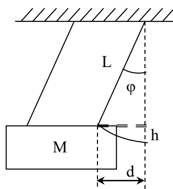
Obr. 2 Balistické kyvadlo
