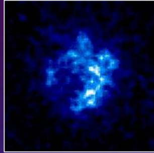
UV
