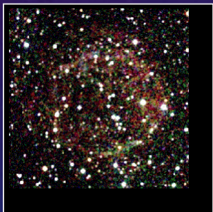
blízká IR
