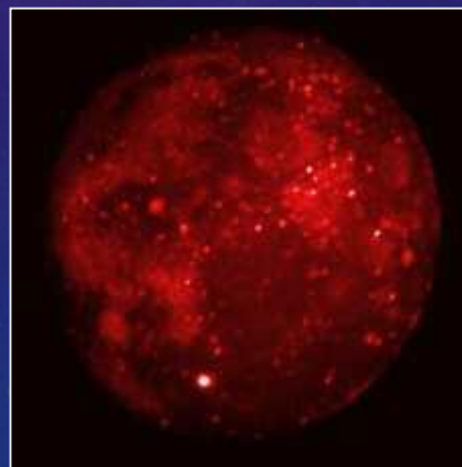
střední IR
