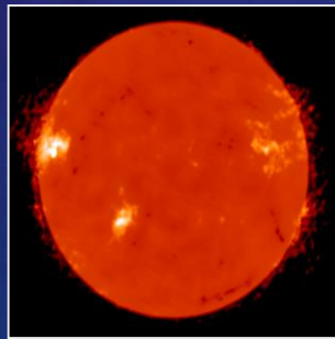
rádiový
