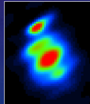
vzdálená IR
