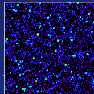
rádiový obor
