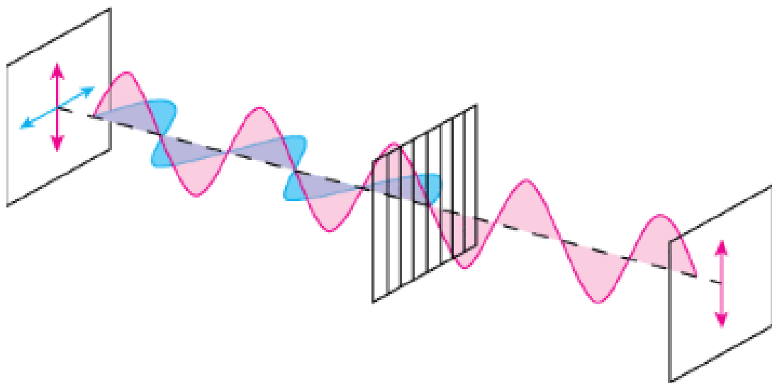
Obr. 1: Vznik polarizovaného světla (zdroj).
