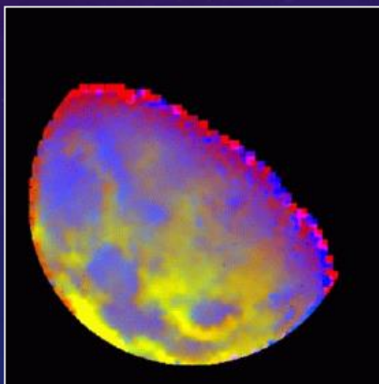
blízké IR
