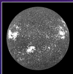
čára K
