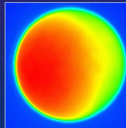
rádiový obor
