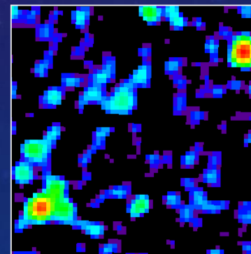
světlo
