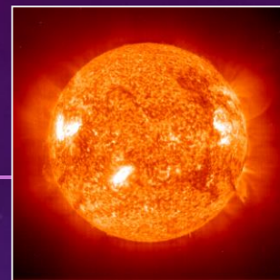
extrémní UV
