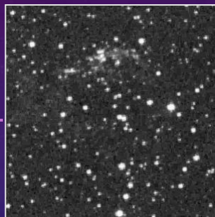
světlo
