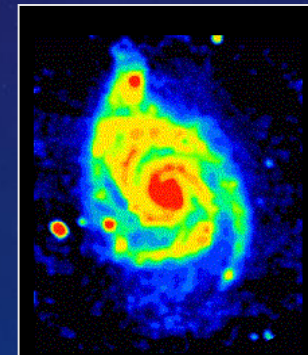
rádiový obor
