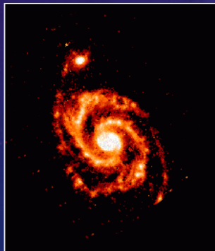
střední IR
