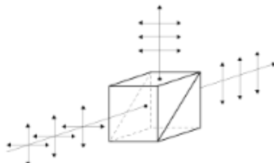
Obr. 2: Vznik polarizace na islandském vápenci (zdroj).
