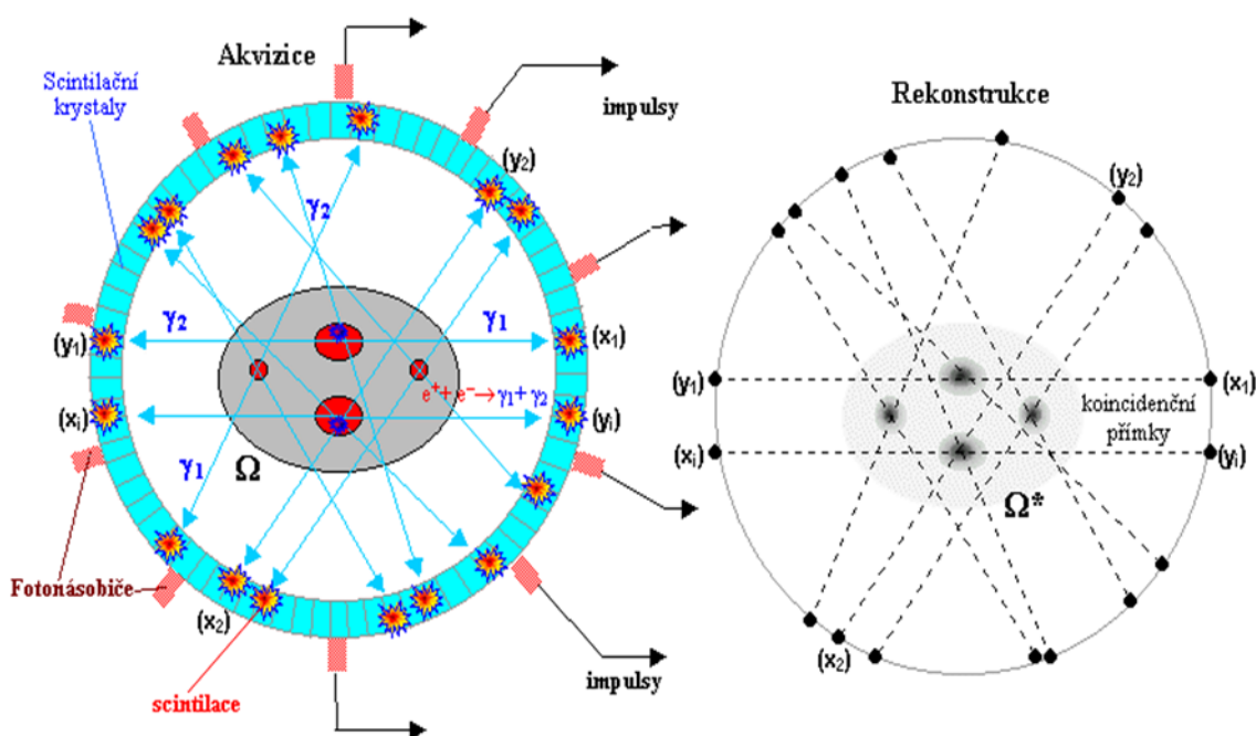
Obrázek 21: Princip PET (podle [17])
