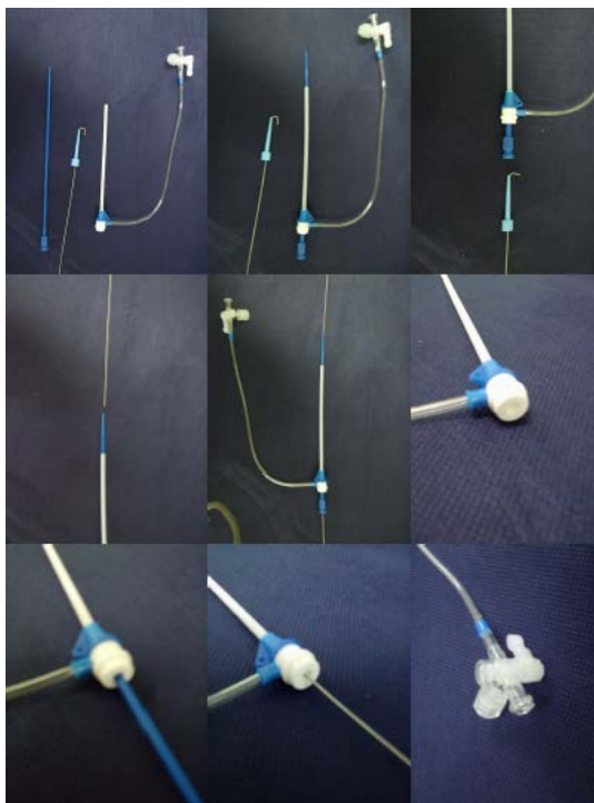
Obrázek 7: Angiografické instrumentárium [18]
