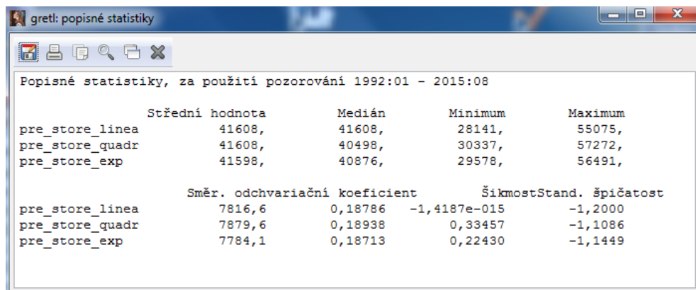
Obr. 3.24: Popisné statistiky 2
