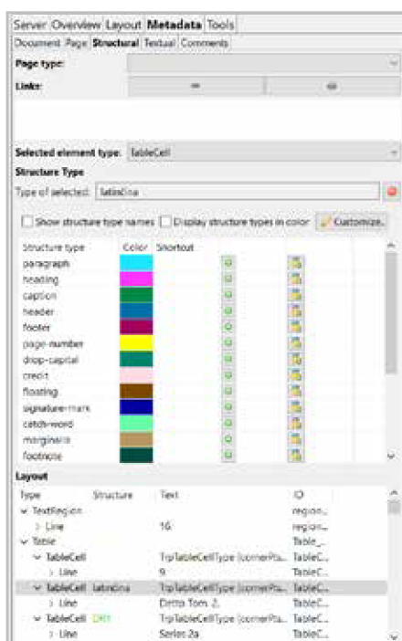
Obrázok 171 Štruktúra záložky Štruktúrne tagy ( Structural )
