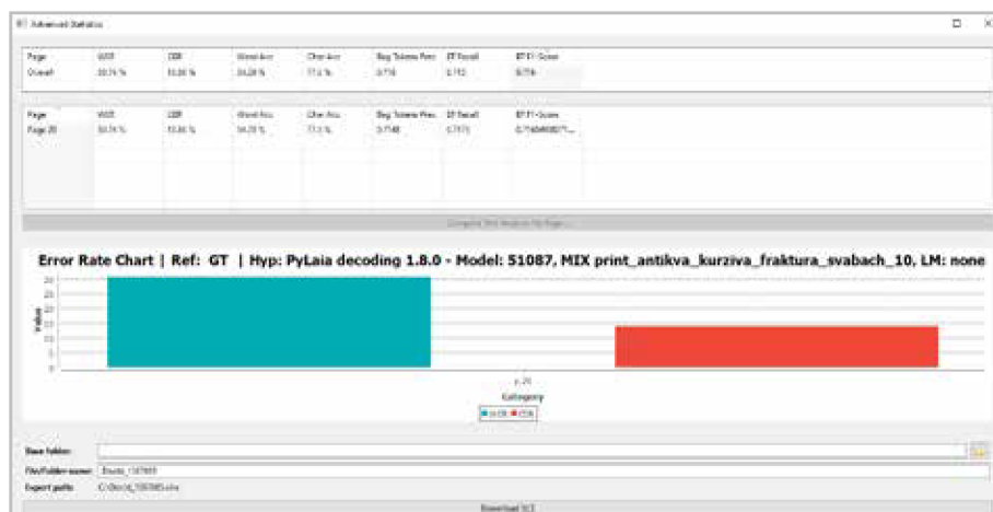
Obrázok 131 Okno rozšírených štatistik
