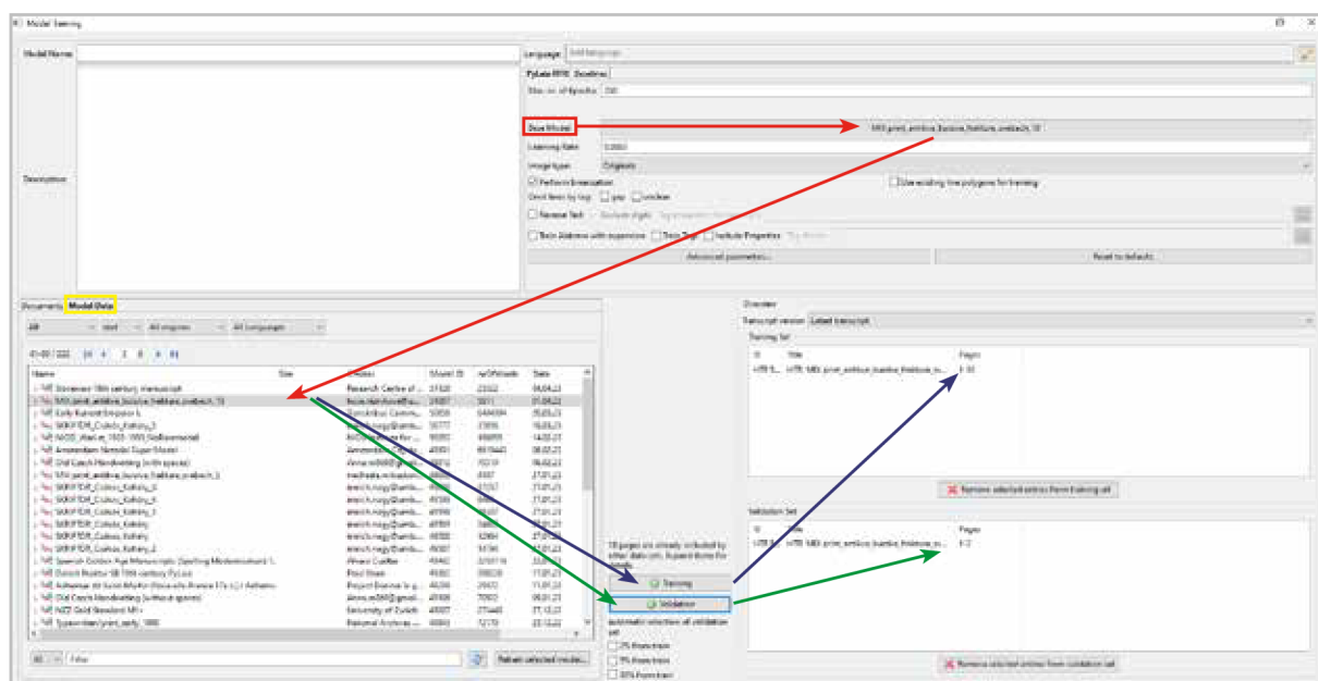
Obrázok 133 Tréňovanie pomocou základného modelu
