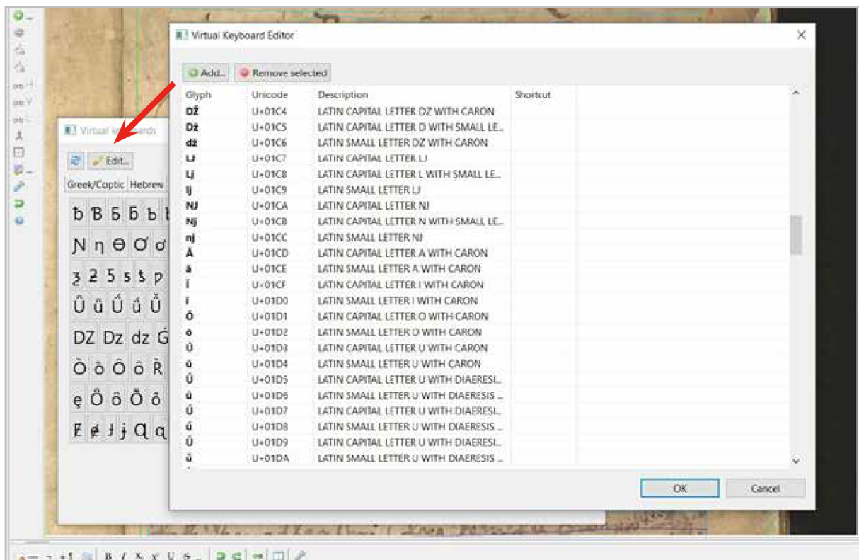
Obrázok 115 Pridávanie glyfov zo sady Unicode
